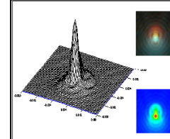
PSF 図
