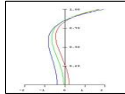
幾何収差図
